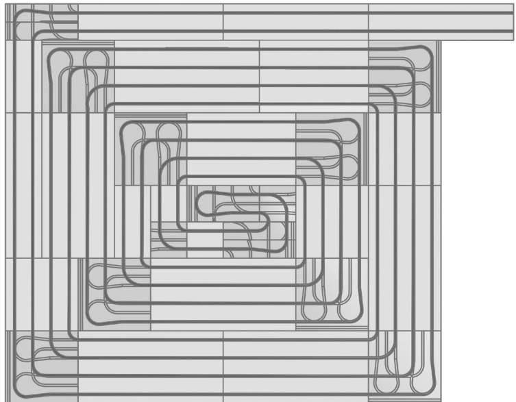
schneckenförmige Rohrführung
